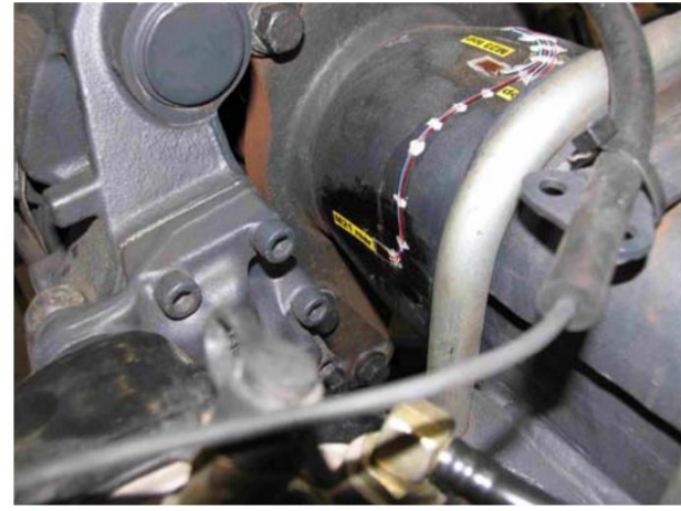
代替六分力的后桥应变测点布置方案
